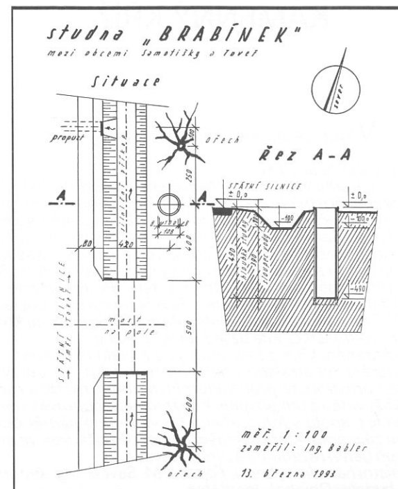
Situace a řez, původní měřítko 1 : 100. Zhotovil Otto Babler.
