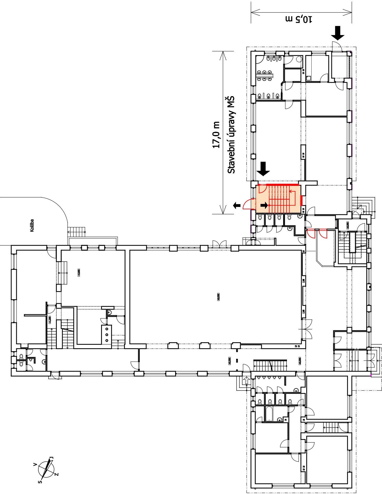
Stavební úpravy a nástavba Matěřské školy Tověř v budově č.p. 18 v Tověři - Půdorys 1NP - M 1:200
